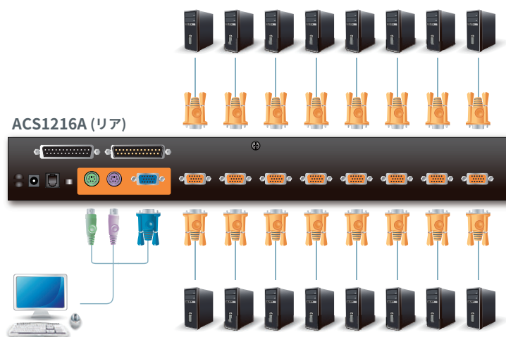
モニター / PS/2マウス / PS/2キーボード
