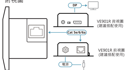
俯視圖
