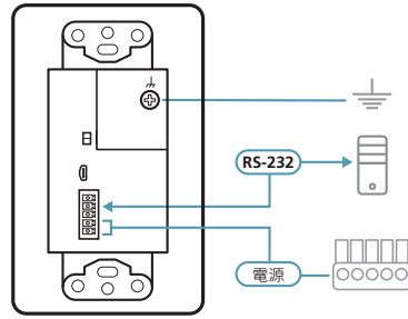
背視圖
