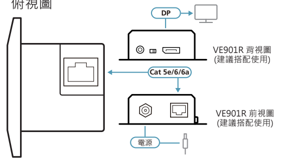
俯視圖
