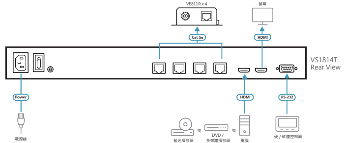
備註：此為VS1814T連線圖，VS1818T與此相同，只是RJ-45母頭連接埠數增加到8個。
